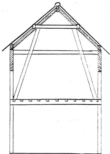
Gebouw na 18de eeuwse verbouwing. Het gearceerde gedeelte is er boven op gekomen.
